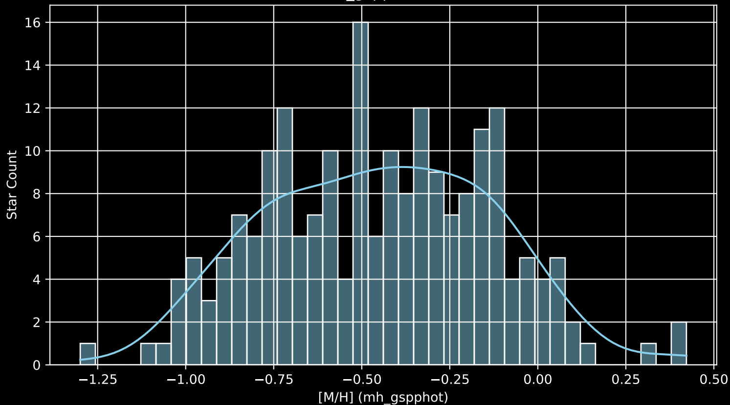
GALAH DR4 Field: [1263] [M/H] (mh_gspphot) (n= 205)
