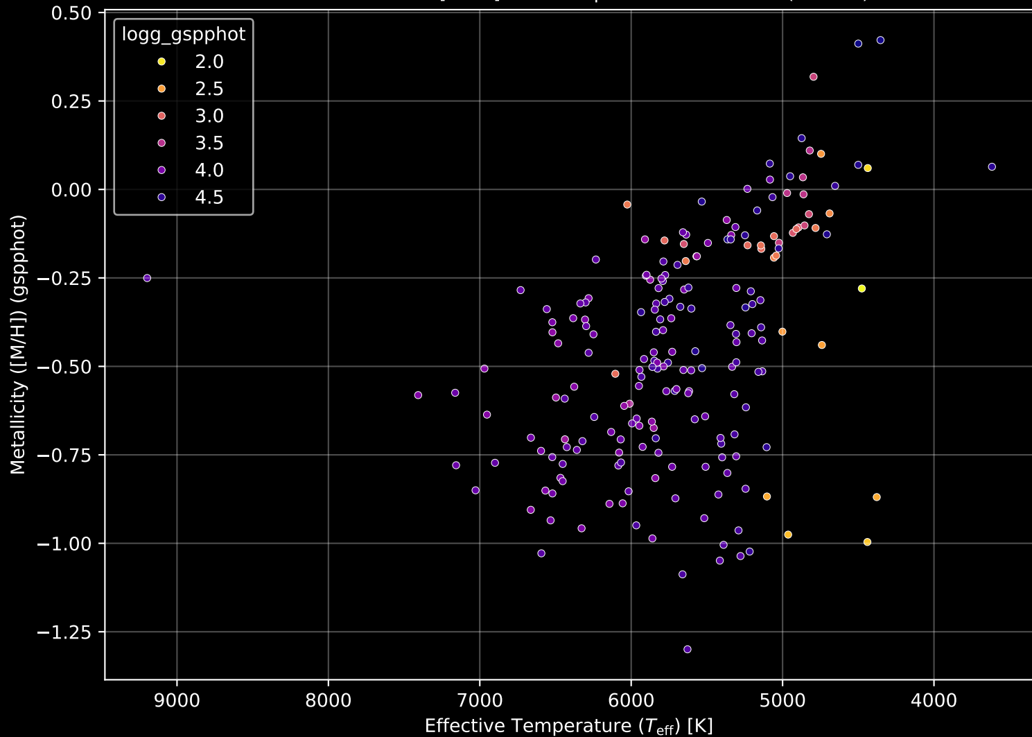
GALAH DR4 Field: [1263] Stellar Population Parameters (n= 205)
