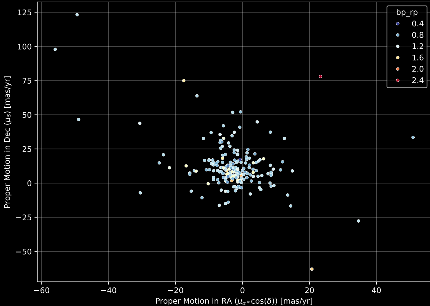
GALAH DR4 Field: [1263] Proper Motion Diagram (n= 205)
