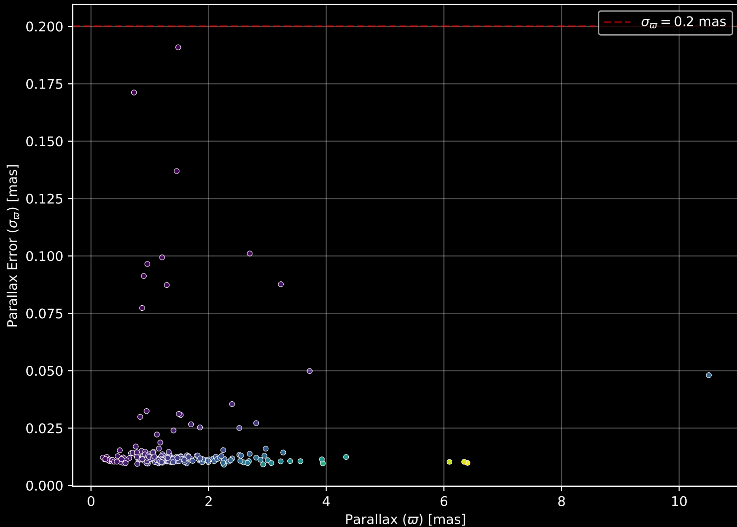
GALAH DR4 Field: [1263] Parallax Quality (n= 205)
